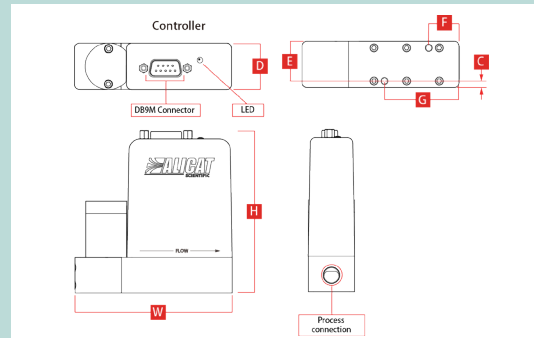
图示为 0-0.5 SCCM 到 0-20 SLPM, 更多量程尺寸请见背面尺寸 / 压损表
